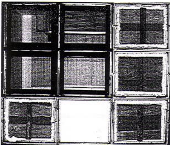
Divisorio posto all'interno della camera climatica, con gli otto pacchetti isolanti di Fibra di legno protetti dalle otto diverse guaine traspiranti, testate.
